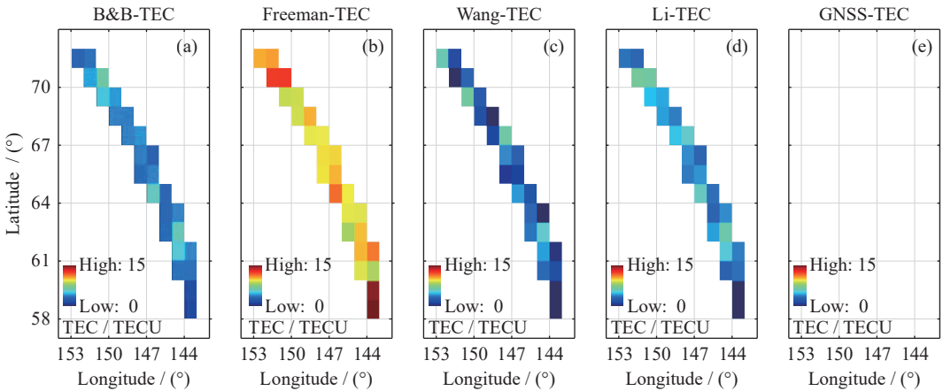
图 3 2007 年 4 月 1 日基于四种 FRA 反演算法的 TEC (a)~(d) 与 GNSS-TEC (e) 对比
