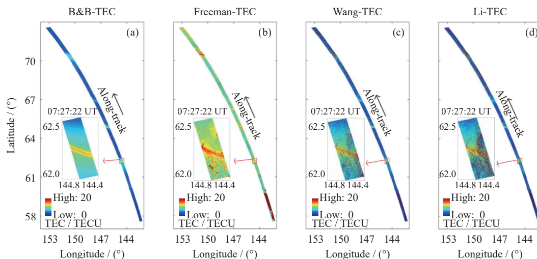
图1 2007年4月1日基于四种FRA反演算法的TEC结果
