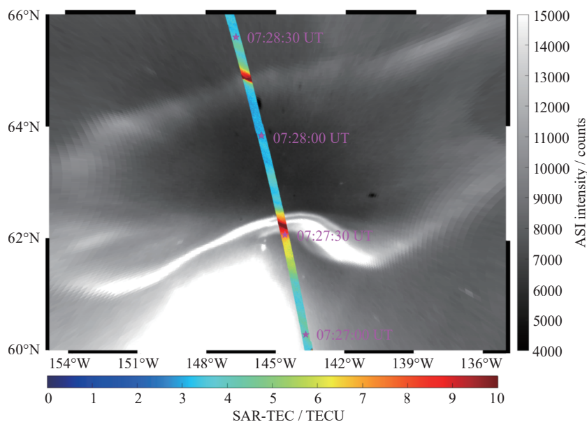
图2 2007年4月1日 THEMIS Gako 台站 ASI 观测与 SAR 反演 TEC 的对比
