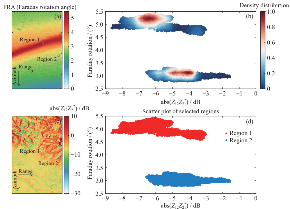
图 4 极光活动时 FRA 与 \text{abs}(Z_{12}Z_{21}^*) 分布及其相关分析
