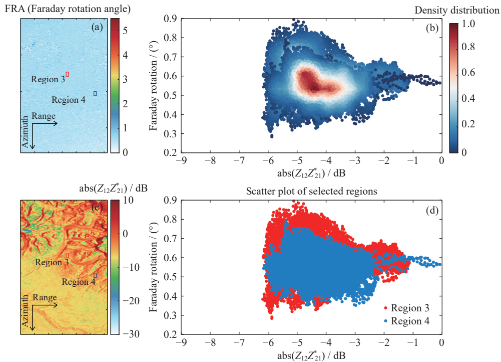
图 5 无极光活动时 FRA 与 \text{abs}(Z_{12}Z_{21}^*) 分布及其相关性分析
