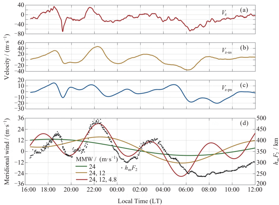
图 6 阿雷西博地区 2015 年 3 月 17 日 16:00 LT 至 3 月 18 日 12:00 LT 期间, 在 380 km 高度处离子垂直飘移速度及分量随时间的变化情况 (修改自文献 [31] )
