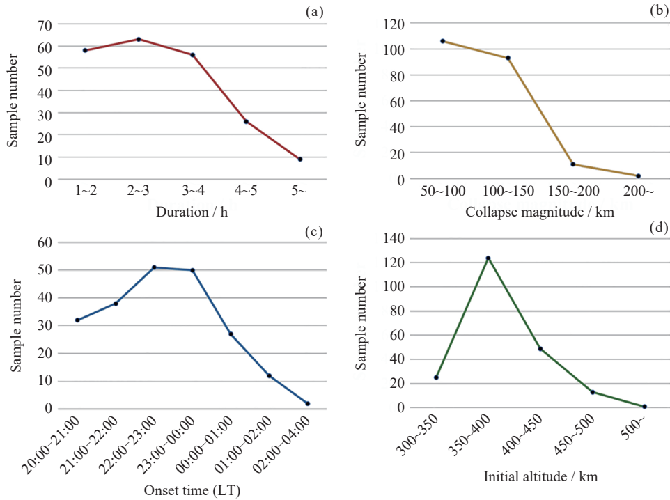
图 2 一次塌陷的统计特征. (a) 持续时间, (b) 塌陷幅度, (c) 起始时间以, (d) 起始高度 (修改自文献 [2])
