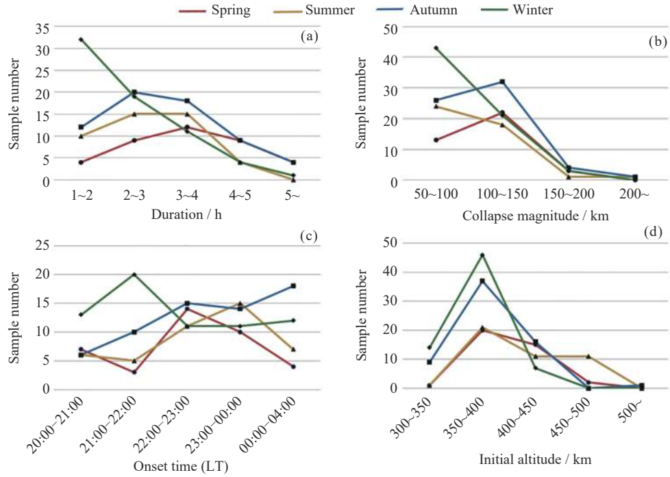
图 3 不同季节条件下一次日夜塌陷统计特征. (a) 持续时间, (b) 塌陷幅度, (c) 起始时间, (d) 起始高度 (修改自文献 [2])
