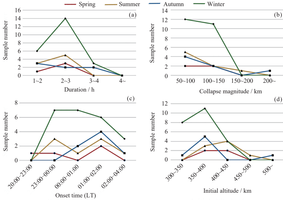
图 5 不同季节条件下二次午夜塌陷统计特征. (a) 持续时间, (b) 塌陷幅度, (c) 起始时间, (d) 起始高度 (修改自文献 [2])
