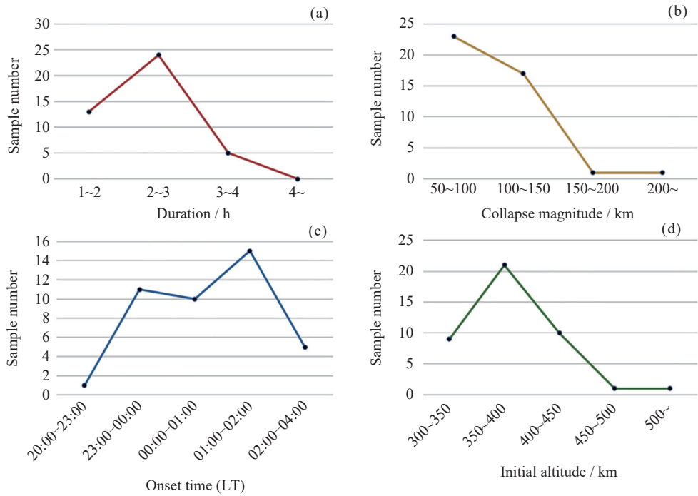
图 4 二次塌陷的统计特征. (a) 持续时间, (b) 塌陷幅度, (c) 起始时间, (d) 起始高度 (修改自文献 [2])
