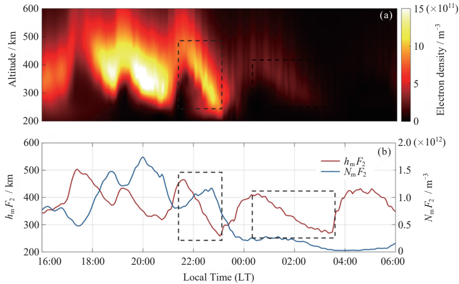
图1 (a) 2011年8月16日16:00 LT至8月17日06:00 LT期间阿雷西博非相干散射雷达观测到的电子密度的高度-时间分布,虚线框标示夜间出现的两次典型午夜塌陷过程.(b) 同一时段F区峰值电子密度( N_m F_2 )及其对应峰值高度( h_m F_2 )的时间演变,用虚线框标出与(a)中对应的午夜塌陷阶段(修改自文献[2])
