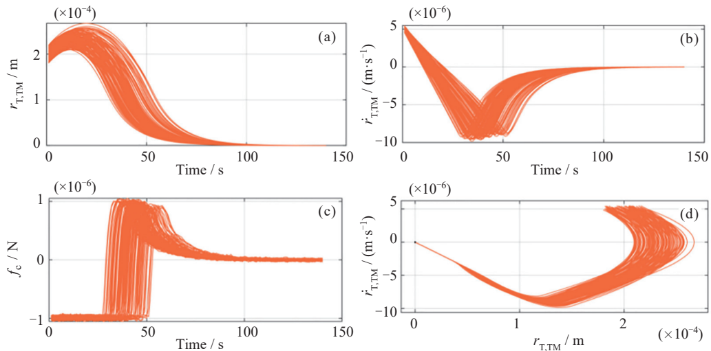
图 21 检验质量相对位移鲁棒性验证
