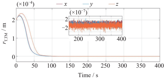
图 9 MPC 线位移
