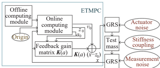
图 5 检验质量捕获控制结构
