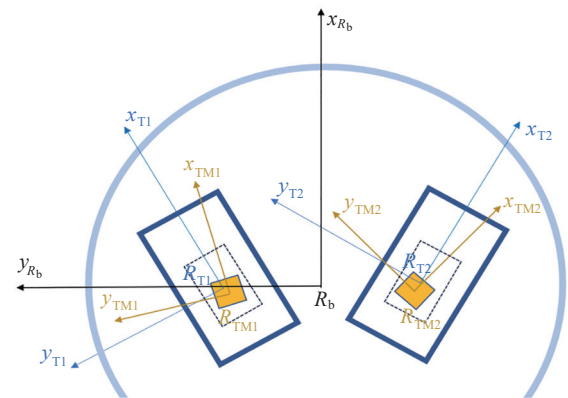
图 2 坐标系定义
