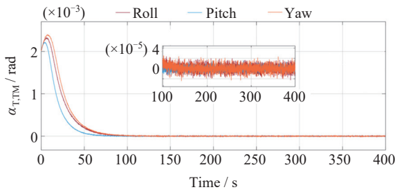
图 11 MPC 角位移
