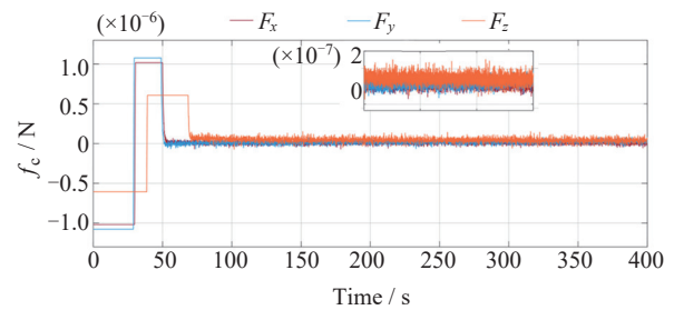
图 18 ETMPC 控制力
