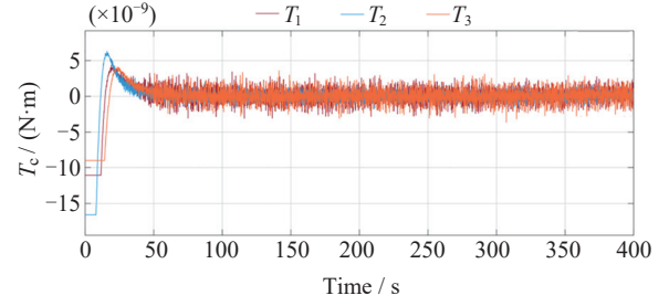
图 12 MPC 控制力矩
