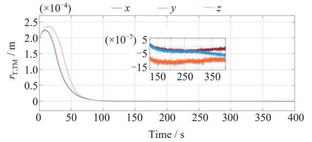
图 13 SMC 线位移
