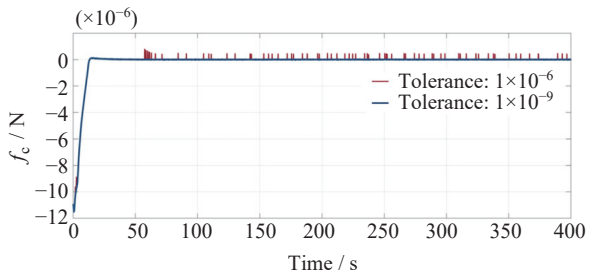
图 7 不同容差 \varepsilon 和 \epsilon 下检验质量捕获控制信号的对比 Fig. 7 Comparison of test mass capture control signals with different tolerances \varepsilon and \epsilon
