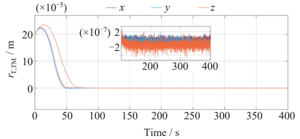
图 17 ETMPC 线位移
