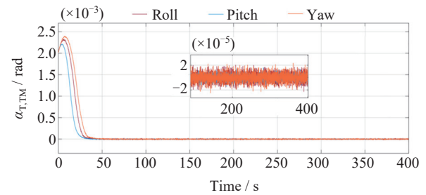
图 19 ETMPC 角位移
