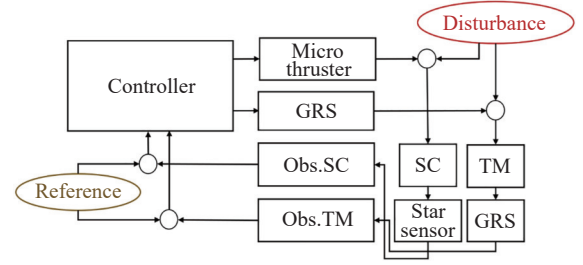
图 3 无拖曳控制系统工作原理
