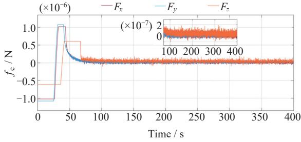
图 10 MPC 控制力
