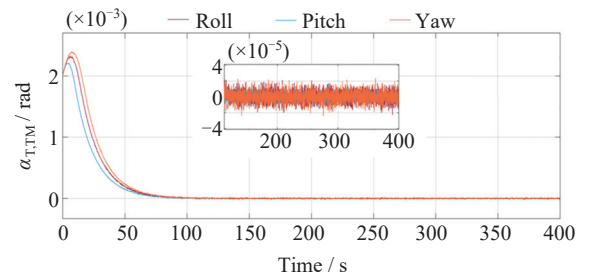
图 15 SMC 角位移
