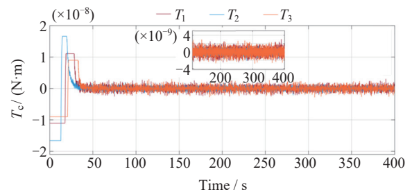
图 20 ETMPC 控制力矩
