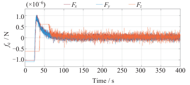
图 14 SMC 控制力
