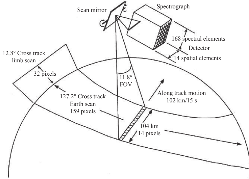
图1 GUVI的扫描示意
