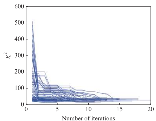
图3 \chi^2 随迭代步数的变化(不同曲线代表不同的反演,每次反演的迭代初值和噪声不同)
