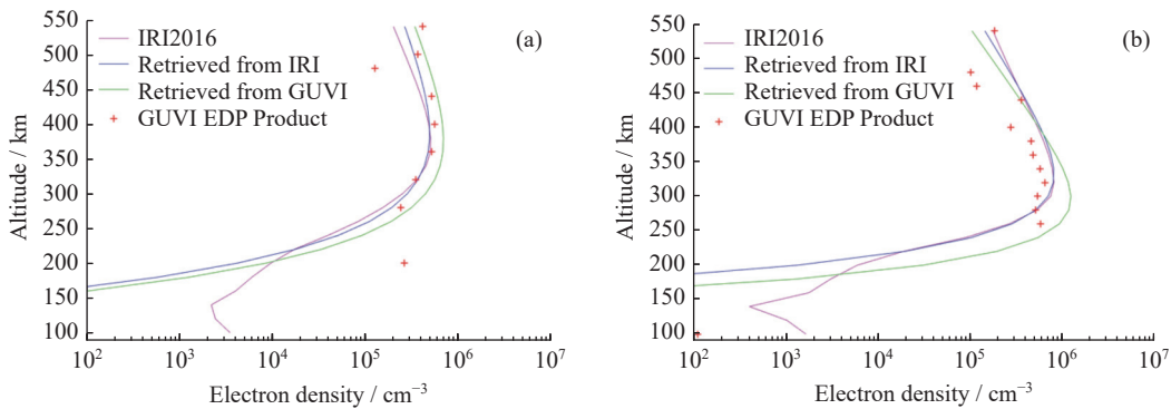
图 7 2002 年 7 月 20 日 (a) 和 2007 年 10 月 4 日 (b) GUVI 135.6 nm 临边观测反演结果典型示例及与相同条件下 IRI2016 模型与 GUVI 数据的 EDP 及基于 IRI2016 模型仿真反演结果的对比
