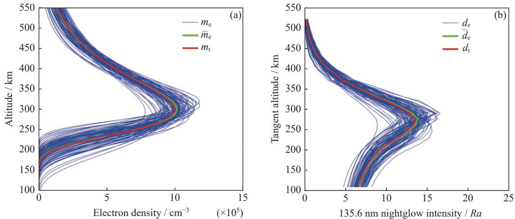
图 5 100 次反演结果及反演结果均值与电离层参数真值对应的电子密度高度 (a) 和 135.6 nm 辐射强度随视线切点高度分布 (b) (每次反演的迭代初值与噪声不同)
