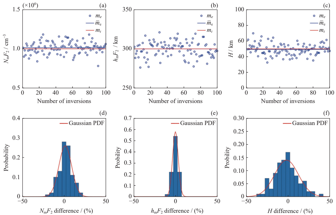
图 4 100 次反演的结果分布及百分比误差的概率密度函数 (PDF) 统计直方图 (每次反演的迭代初值和噪声不同)
