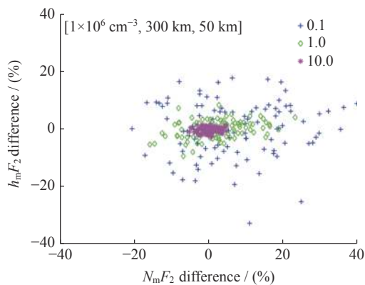
图 6 三种仪器响应度情况下的 N_m F_2 和 h_m F_2 反演百分比误差对比
