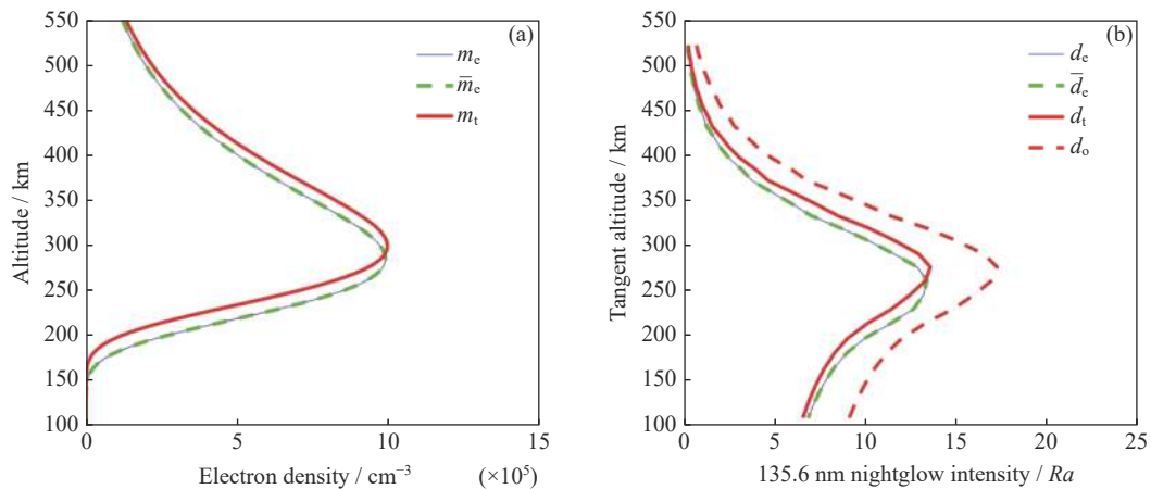
图2 10次反演结果及反演结果均值与电离层参数真值对应的电子密度高度(a)和135.6 nm辐射强度随视线切点高度的分布(b)。10次反演叠加的噪声相同但迭代初值不同
