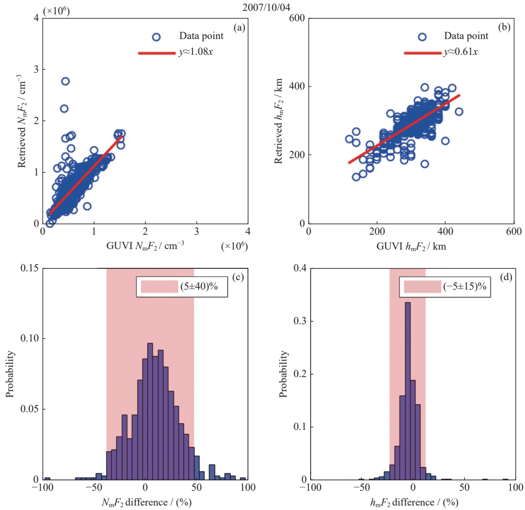
图 9 2007 年 10 月 4 日的观测数据反演获得的电离层参数与 GUVI 数据电离层参数的比较
