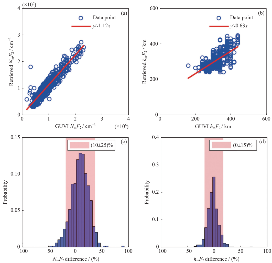
图 8 2002 年 7 月 20 日的观测数据反演获得的电离层参数与 GUVI 数据电离层参数的比较
