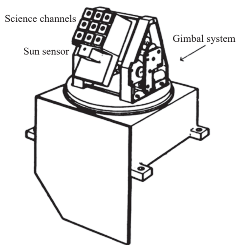
图 5 POAM 系列仪器光学头部组件
