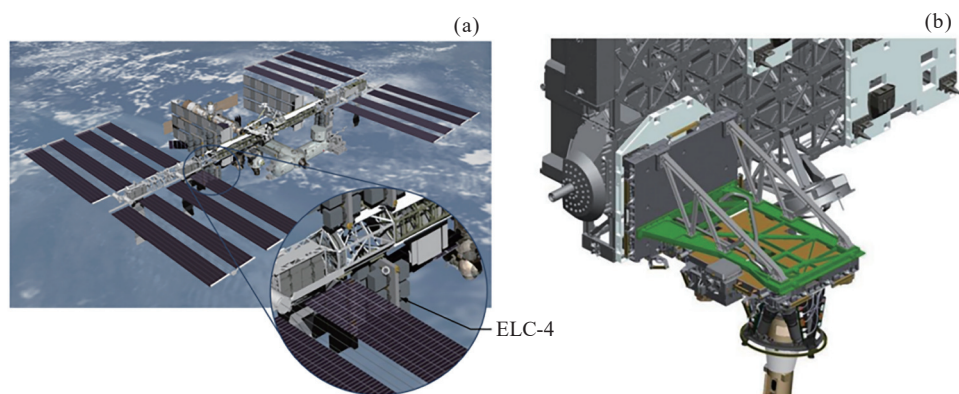
图 16 搭载在国际空间站 ELC-4 区域 (a) 的 SAGE III 掩日仪 (b) Fig. 16 SAGE III solar occultation instrument (b) mounted on the International Space Station's ELC-4 platform (a)
