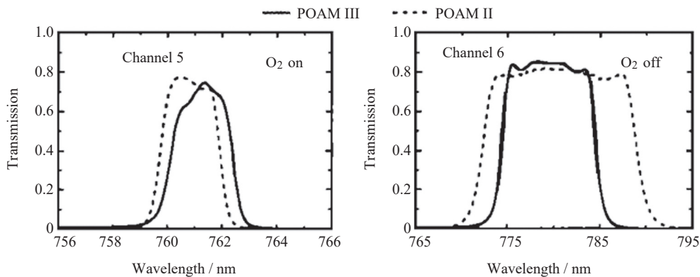
图 6 POAM 氧气探测通道波段设计
