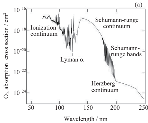
图 2 (a) 氧分子吸收截面, 150 nm 紫外氧气 SR 连续吸收带, (b) 受温度影响较大的 760 nm 红外氧气吸收 A 带
