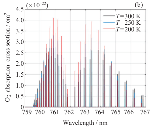
图 2 (a) 氧分子吸收截面, 150 nm 紫外氧气 SR 连续吸收带, (b) 受温度影响较大的 760 nm 红外氧气吸收 A 带
