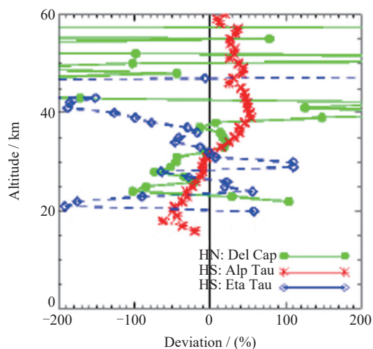
图 11 GOMOS 掩星探测结果与 POAM 结果对比
