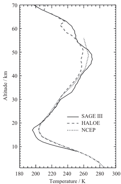
图 18 典型 SAGE III 温度探测结果对比 Fig. 18 Comparison of a typical SAGE III temperature retrieval results
