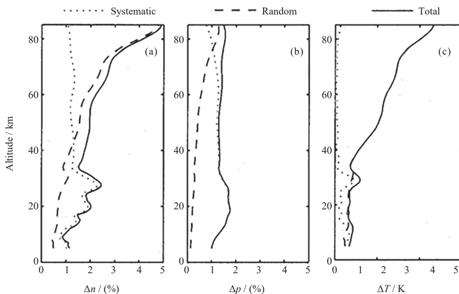
图 15 掩星编号 ss3004 的预期系统、随机和总误差
