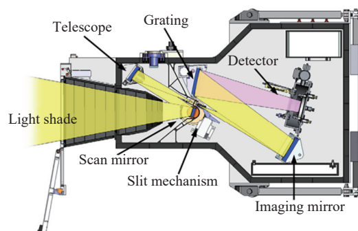
图 23 GOLD 仪器光路设计
