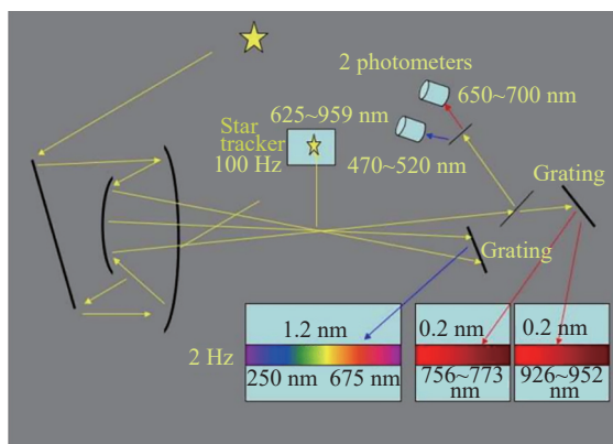
图 10 GOMOS 光路
