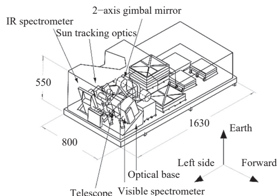
图7 ILAS仪器平面结果(单位:mm)
