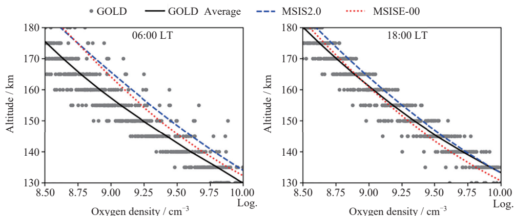
图 24 GOLD 观测的 2019—2021 冬至日 25°S—25°N 氧气密度曲线
