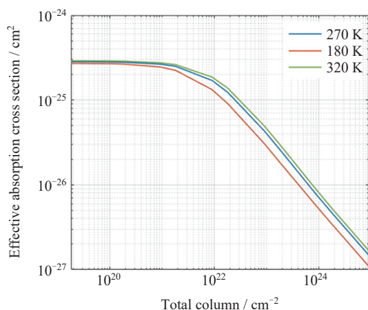
图 3 不同分子数对应有有效吸收截面
