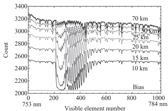
图8 一次典型的切线海拔ILAS掩日红外光谱测量
