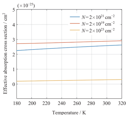
图 4 有效吸收截面随温度的变化
