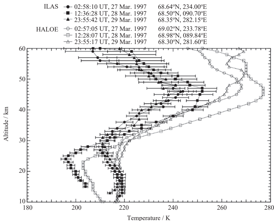
图 9 通过 ILAS 探测氧气得到的温度剖面与 HALOE 结果对比
