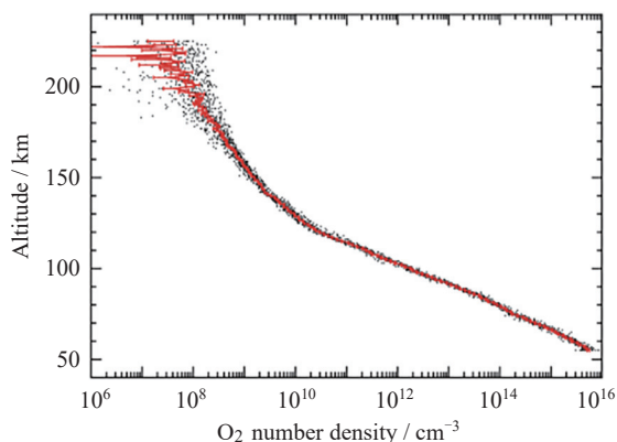
图 22 从 UVISI 掩星中反演得到的氧气密度剖面 (黑点表示单个剖面, 红线表示加权平均剖面及 \pm 1 标准差范围)
