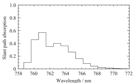
图 17 SAGE III 以 1 nm 分辨率探测切点 海拔 20 km 吸收光谱
