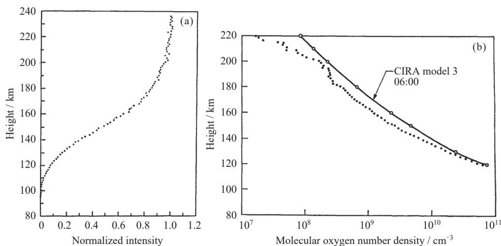
图 20 OAO-2 探测到的一次掩星事件归一化光强 (a) 及其氧气密度反演结果 (b)
