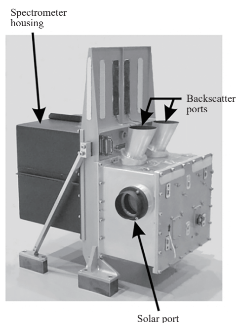
图 13 MAESTRO 掩日仪器照片
