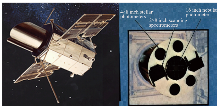
图 19 OAO-2 卫星平台 (a) 与紫外望远镜系统 (b)
