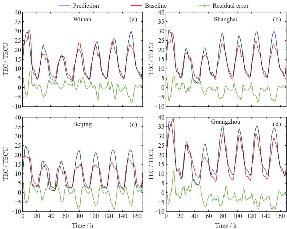
图 5 地磁活跃期间得到的 7 天预测值与真实值
