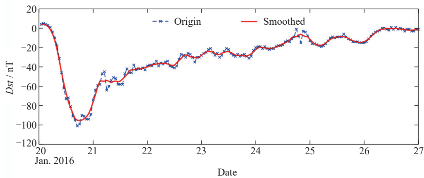
图 4 2016 年 1 月 20—26 日连续 7 天的 Dst 指数
