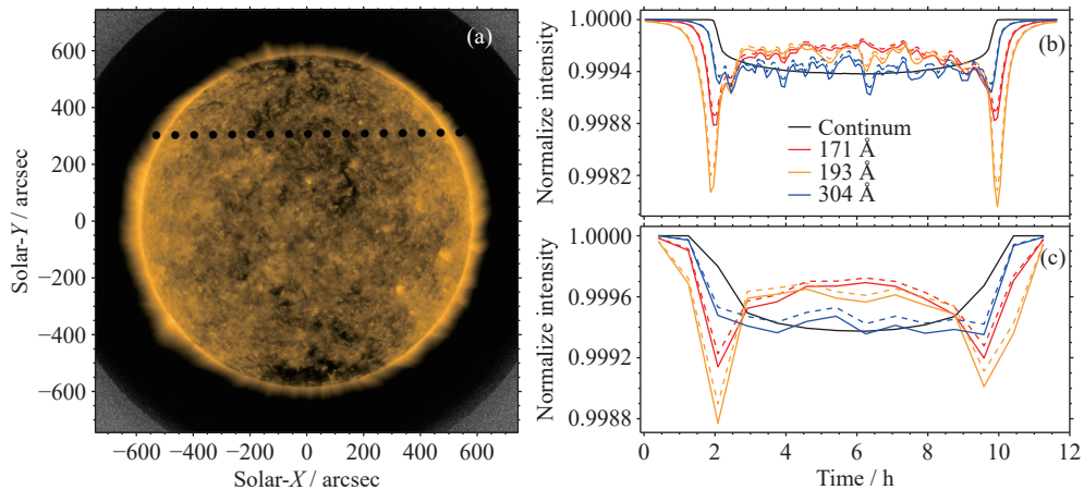
图 6 夸父二号观测地球凌日过程的模拟结果. (a) 根据卫星轨道计算得到的地球凌日过程中投影到太阳表面的位置及投影半径, (b) 凌日过程中极紫外 171, 193 和 304 Å 及可见光波段的光变曲线, (c) 曝光时间提高至 50 min 时得到的光变曲线
