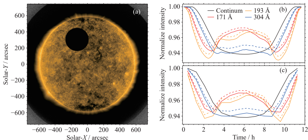
图 7 与图 6 类似但将图 6 中地球及其大气放大 10 倍以后的结果
