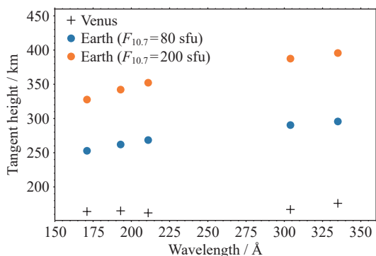
图 5 金星和地球掩日观测时在 171, 193, 211, 304 和 335 Å 波段的大气遮挡高度 (透过率为 50% 时的切向高度).
