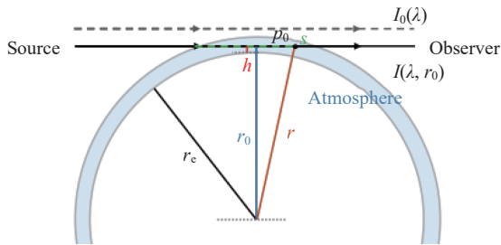
图 2 掩星观测
