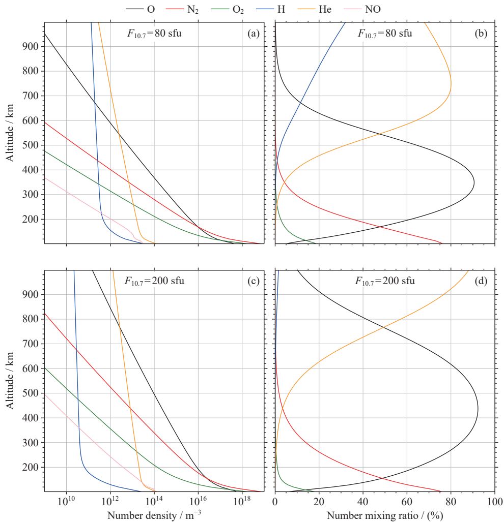
图 3 NRLMSIS2.1 经验大气模型在赤道附近冬季 06:00 LT 条件下的垂直廓线. (a)(c) 为氧分子、氮分子、氧原子、氢原子、氦原子以及一氧化氮分子为数密度随高度的变化廓线, (b)(d) 给出了这些原子和分子为数混合比随高度的分布, (a)(b) 对应 F_{10.7} = 80 sfu 的情况, (c)(d) 对应 F_{10.7} = 200 sfu 的情况
