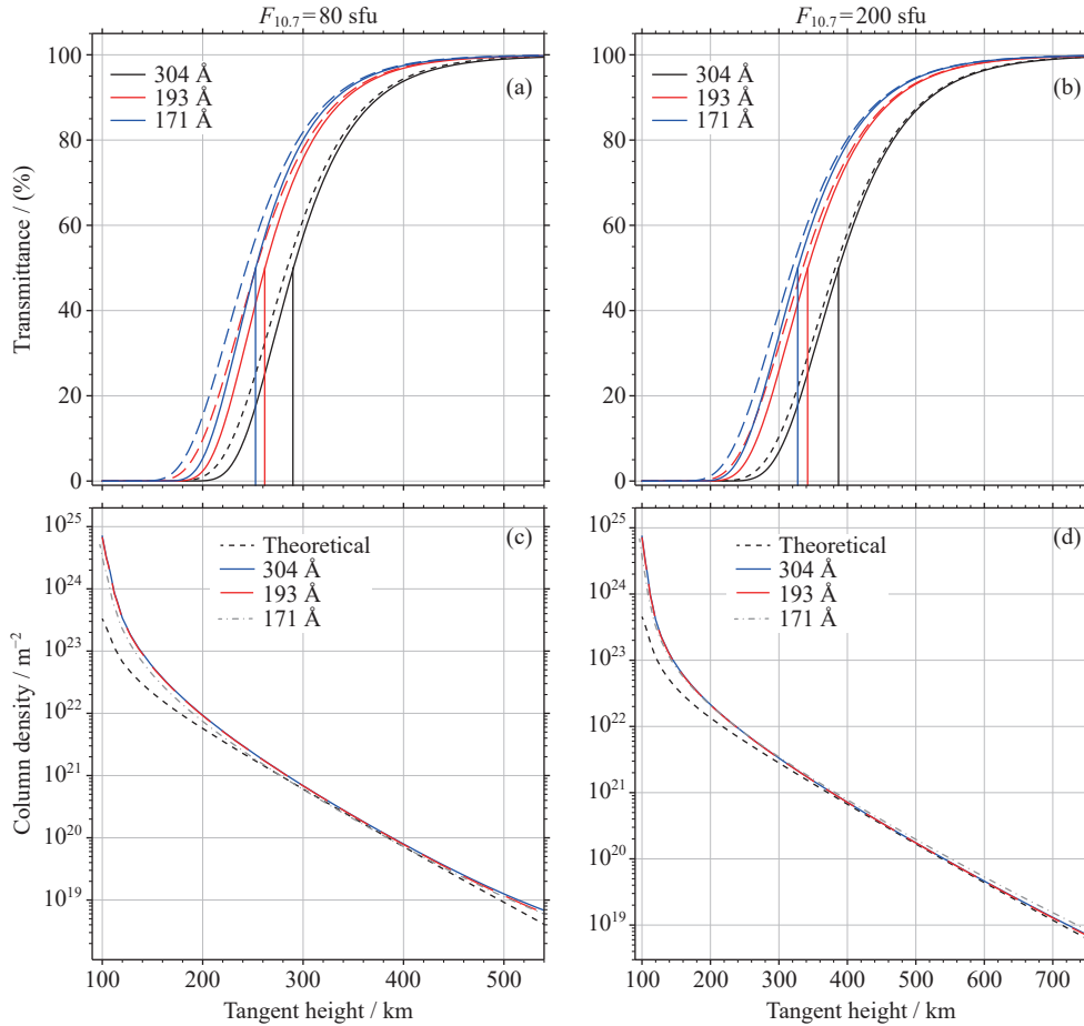
图 4 地球大气对极紫外辐射的正演透过率与反演柱密度. (a)(b) 在 F_{10.7} = 80 sfu 和 200 sfu 的条件下, 正演计算得到的极紫外 171, 193, 304 Å 三个波段的辐射透过率, (c)(d) 基于上述透过率反演得到的氧原子柱密度随高度的分布
