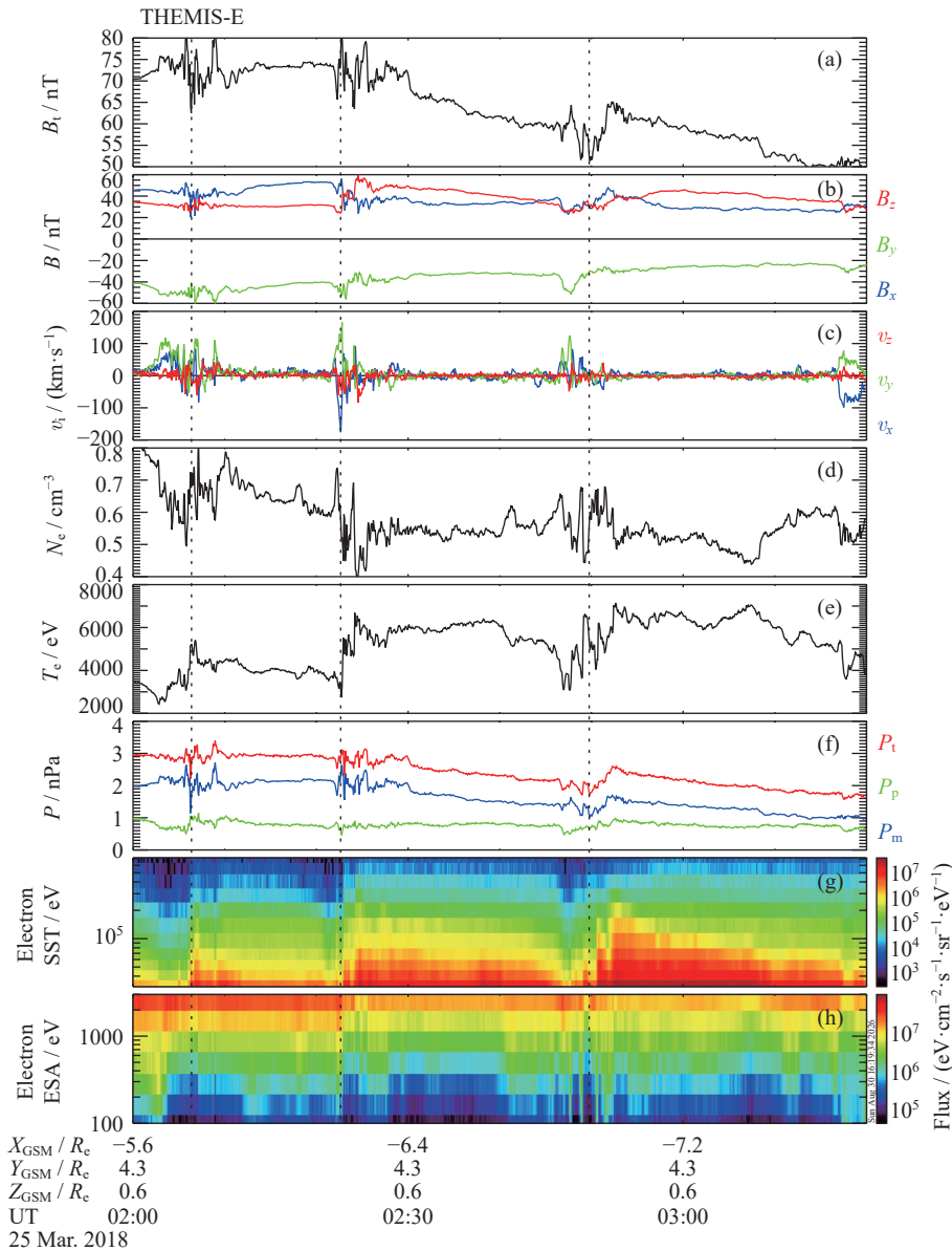
图9 2018年3月25日02:00–03:20 UT期间 THEMIS-E 的观测结果
