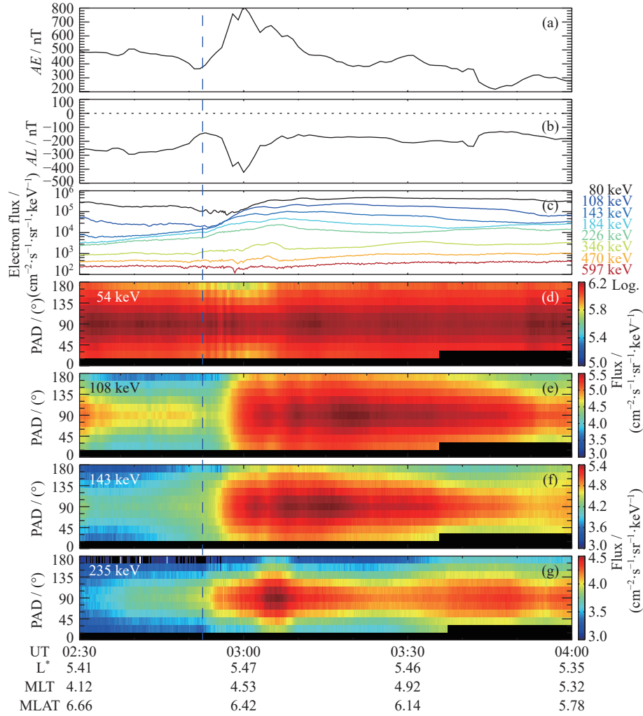
图 15 2014 年 9 月 24 日 02:30–04:00 UT 期间范艾伦探测器 A 的观测结果
