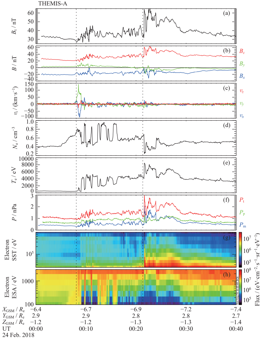
图 1 2018 年 2 月 24 日 00:00—00:40 UT 期间 THEMIS-A 的观测结果. (a)(b) 由磁通门磁力计 (FGM) 测量的总磁场 ( B_t ) 和磁场 ( B ), (c)~(e) 由静电分析仪 (ESA) 和固态望远镜 (SST) 测量的离子速度 ( v_i )、电子密度 ( N_e ) 和温度 ( T_e ), (f) 磁场压强 P_m (蓝线)、等离子体压强 (离子与电子之和) P_{th} (绿线) 和总压强 P_t (红线), (g)(h) 由 SST 和 ESA 仪器观测得到的 0.1~700 keV 电子能谱
