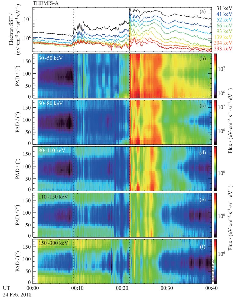
图 2 2018 年 2 月 24 日 00:00—00:40 UT THEMIS-A 电子观测结果. (a) SST 测量的电子全向微分通量, (b)~(f) SST 能量范围 (30~300 keV) 内电子通量随投掷角的变化
