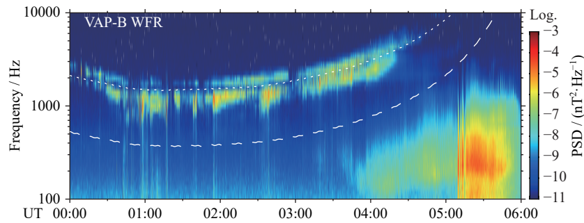
图 4 2018 年 2 月 24 日 00:00–06:00 UT 期间范艾伦探测器 B 上 EMFISIS 测量的磁场谱
