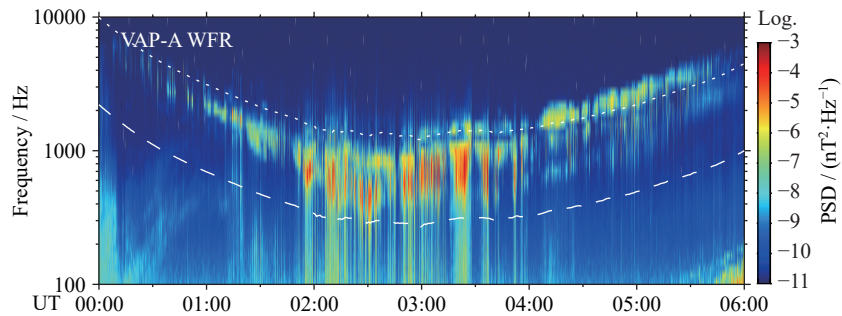
图 16 范艾伦探测器 B 上 EMFISIS 在 2014 年 9 月 24 日 00:00–06:00 UT 测量的磁场谱
