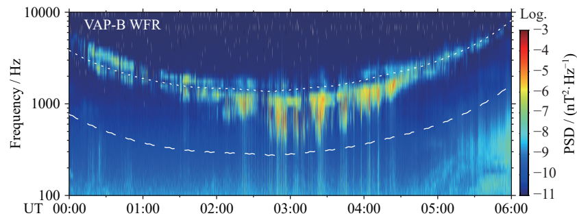
图 12 2018 年 3 月 25 日 00:00–06:00 UT 范艾伦探测器 B 上 EMFISIS 仪器测量的磁场谱
