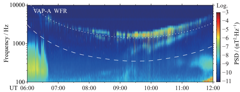
图 8 2018 年 3 月 26 日 06:00–12:00 UT 范艾伦探测器 A 上 EMFISIS 测量的磁场谱
