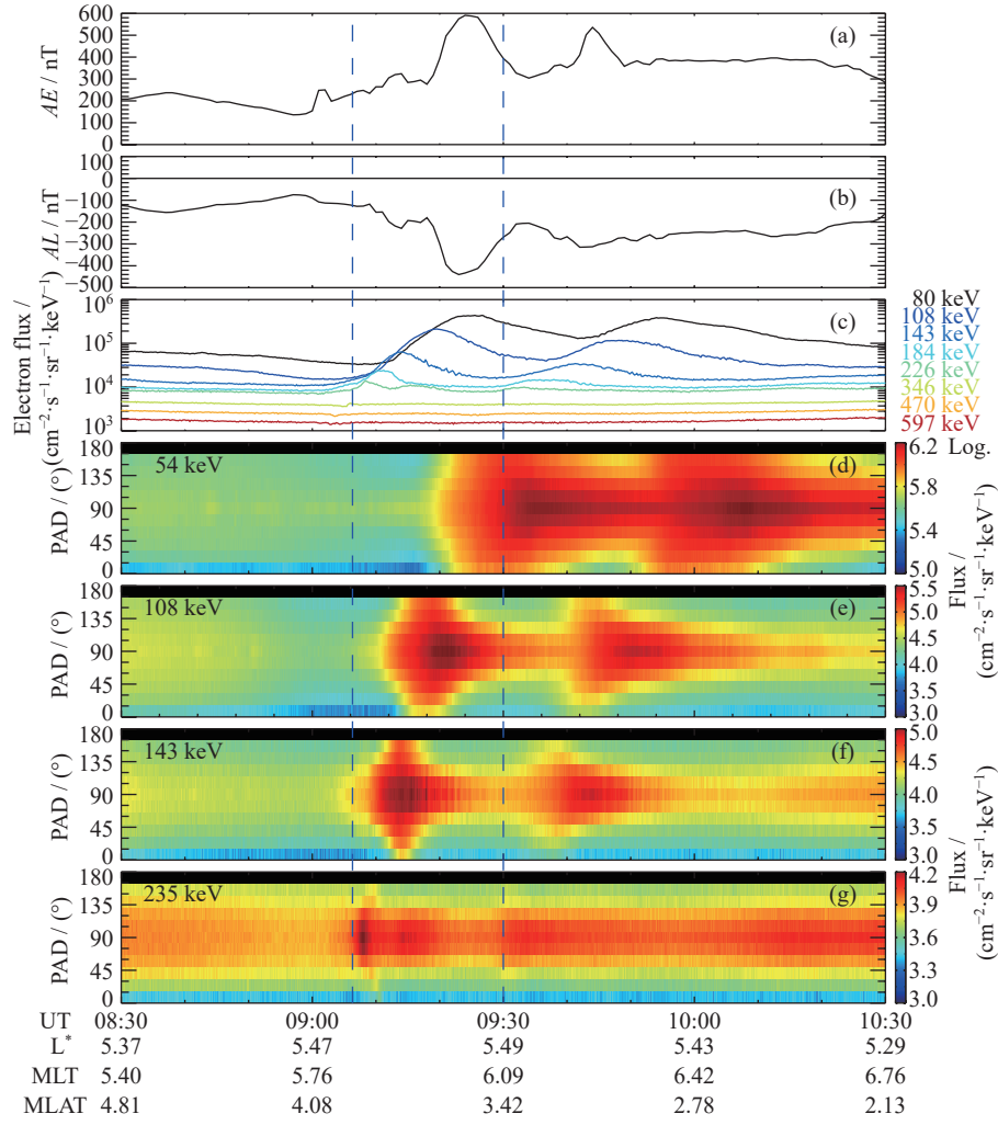
图 7 2018 年 3 月 26 日 08:30–10:30 UT 期间范艾伦探测器 A 的观测结果
