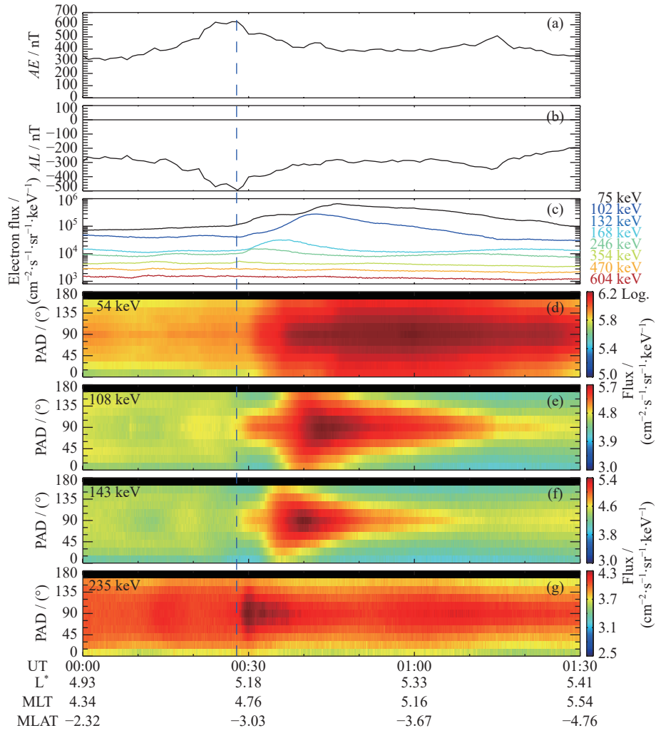
图 3 2018 年 2 月 24 日 00:00–01:30 UT 期间范艾伦探测器 B 的观测结果. (a)(b) 地磁指数 ( AE 与 AL ); (c)~(g) MagEIS 测量的能量电子微分通量、不同能量 (54~235 keV) 电子的投掷角分布
