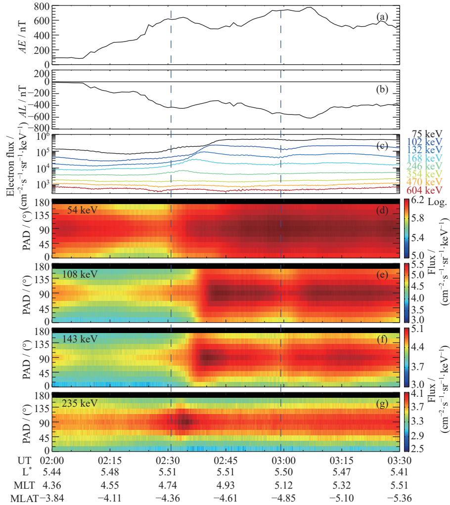
图 11 2018 年 3 月 25 日 02:00–03:30 UT 期间范艾伦探测器 B 的观测结果
