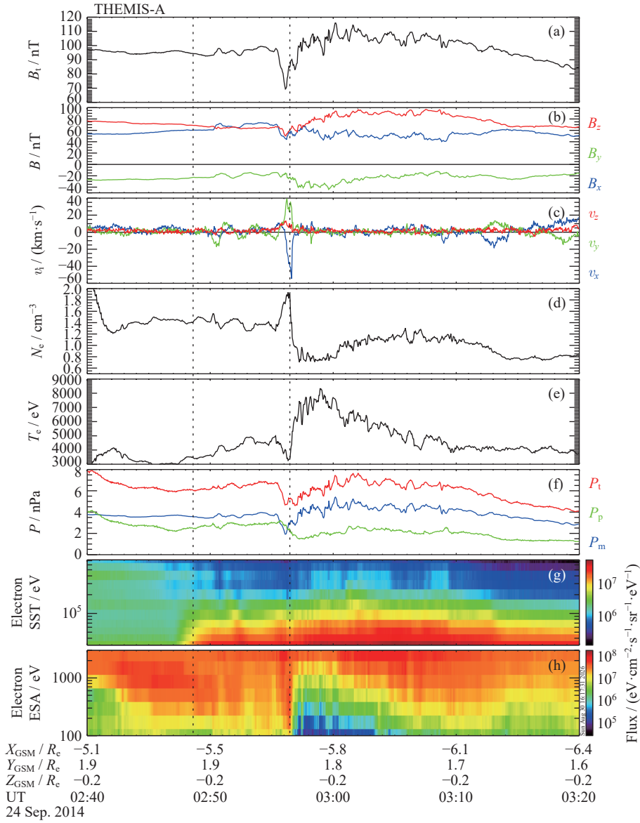
图 13 2014 年 9 月 24 日 02:40–03:20 UT 期间 THEMIS-A 的观测结果
