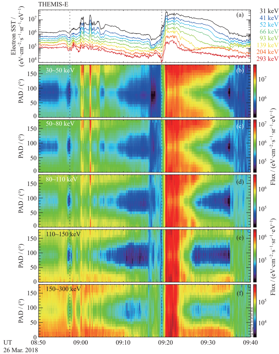
图6 2018年3月26日08:50–09:40 UT期间 THEMIS-E 的电子观测结果
