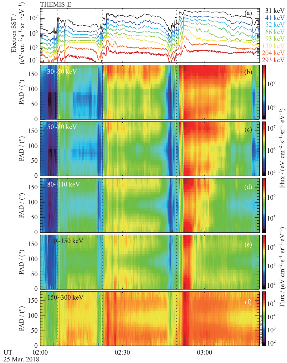
图 10 2018 年 3 月 25 日 02:00—03:20 UT 期间 THEMIS-E 的电子观测结果
