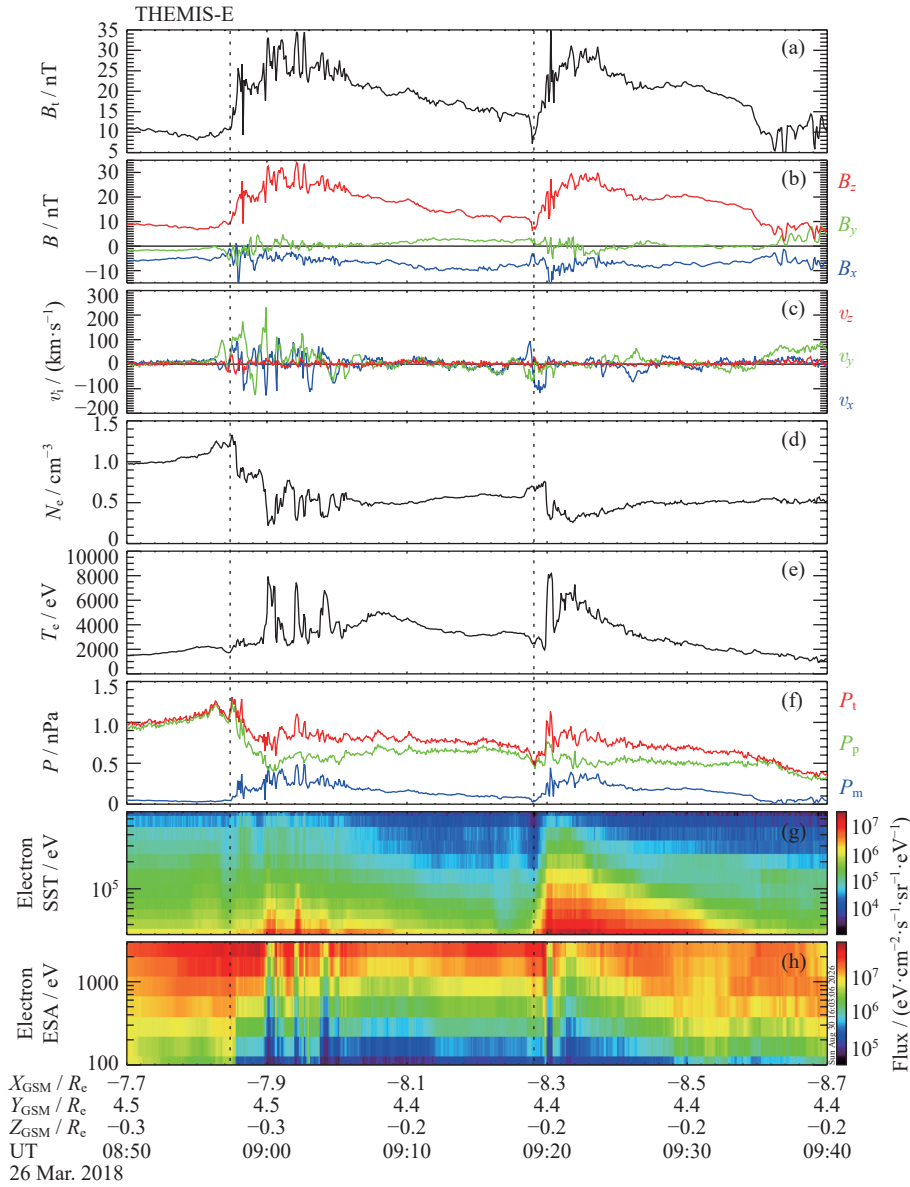
图 5 2018 年 3 月 26 日 08:50—09:40 UT 期间 THEMIS-E 的观测结果
