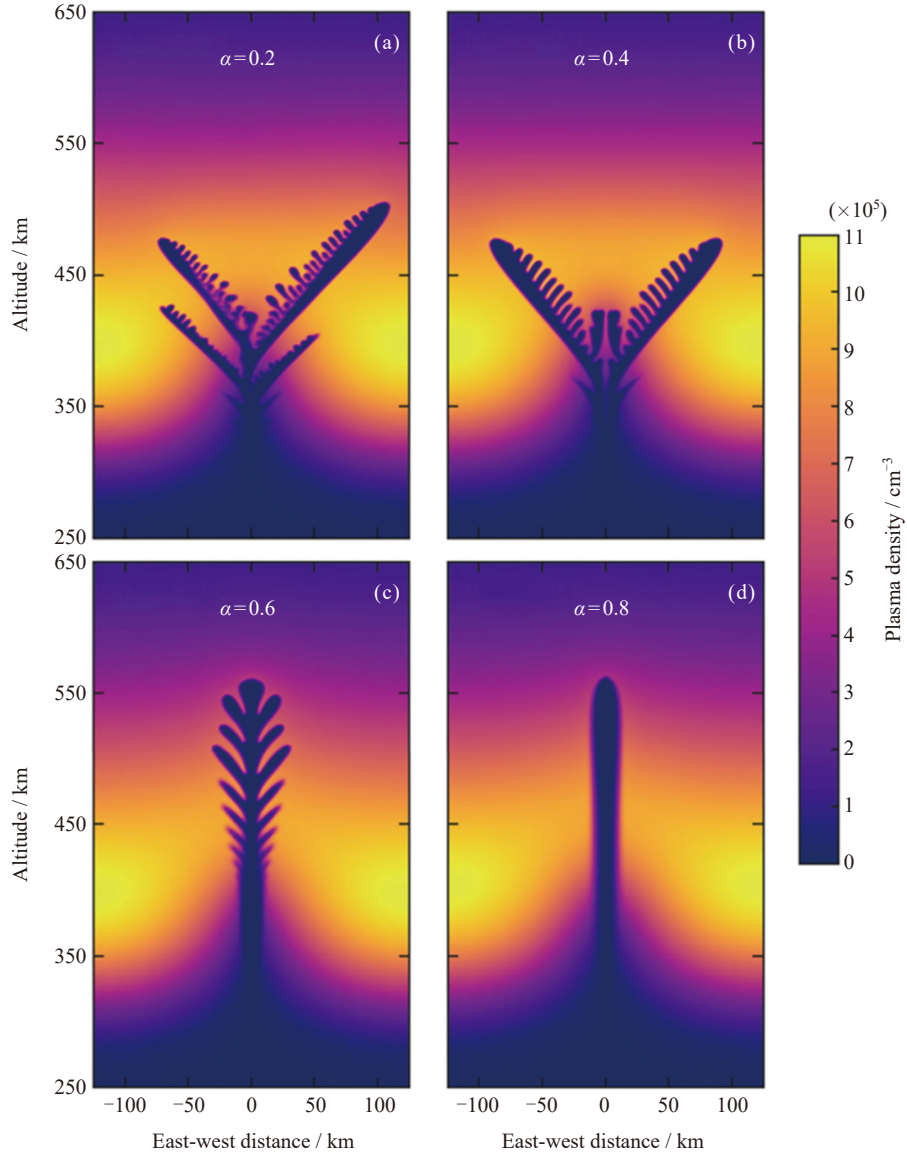
图 2 采用不同 PDM 参数 \alpha 取值的电离层不规则体二维模拟结果 [13]
