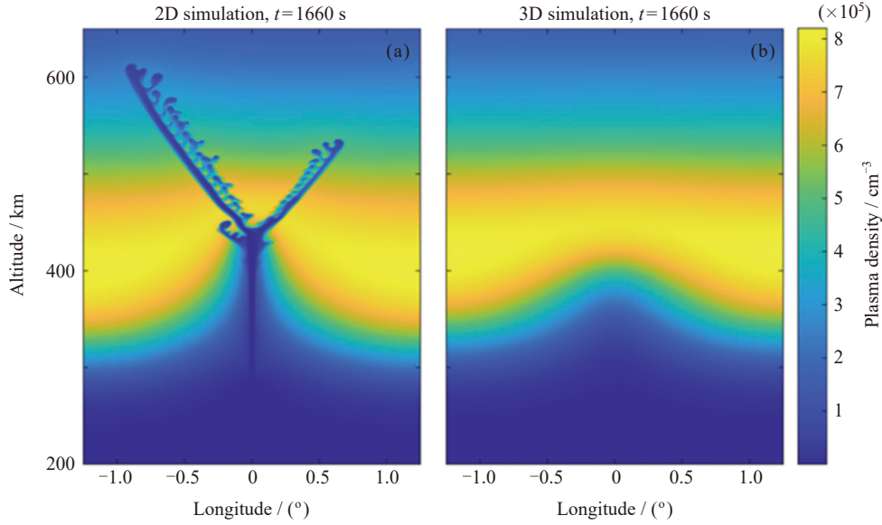
图 4 t = 1660 s 时刻二维和三维理论模式模拟的赤道面内低纬电离层不规则体等离子体密度分布 [15]
