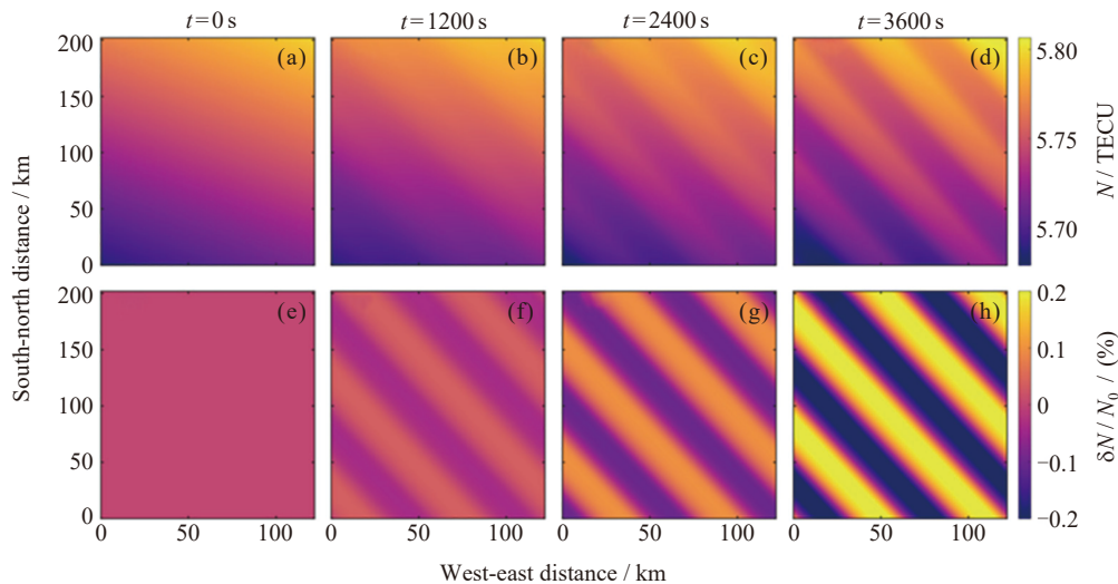
图 5 地磁平静时期 t=0 s, 1200 s, 2400 s 和 3600 s 时, 积分等离子体密度 N (a)~(d) 及扰动等离子体密度 \delta N 相对于背景积分等离子体密度 N_0 的百分比 (e)~(h) [17]
