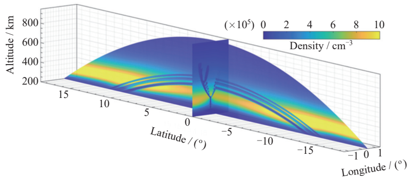
图 3 t = 3500 s 时刻三维模拟得到的等离子体密度在经度面、赤道面与 \pm 10^\circ 纬度面上的分布 [15]
