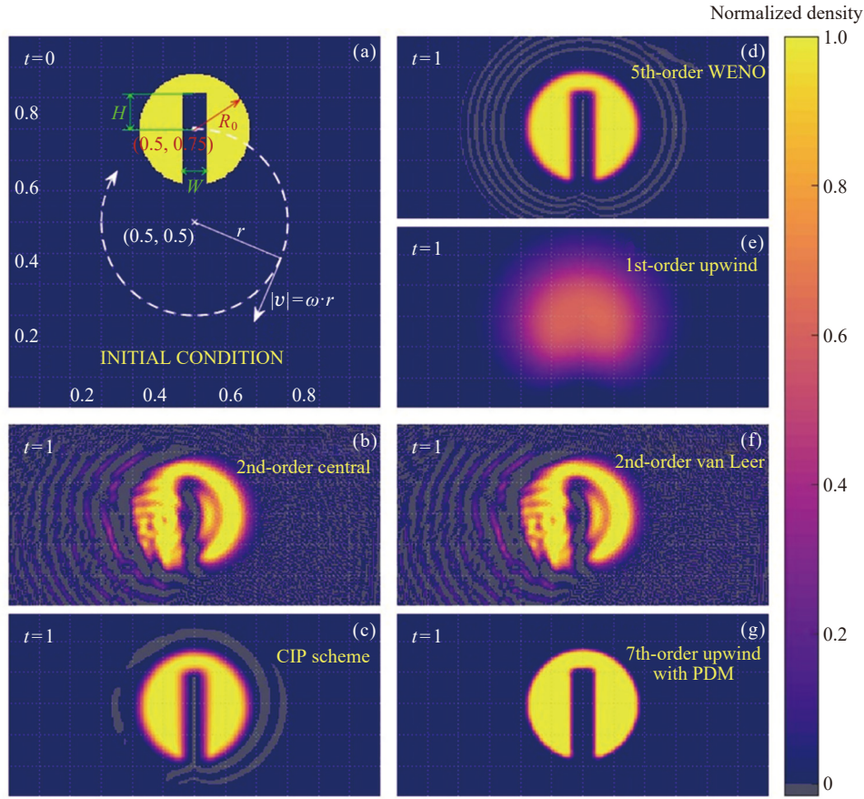
图 1 环形对流测试的初始条件和 t=1 时使用不同对流方法的结果 [13] . (a) t=0 时 256 \times 256 个笛卡尔网格上的开槽圆盘状初始密度分布及绕模拟区域中心顺时针旋转的速度场, (b)~(g) t=1 时 (绕中心旋转一周) 使用不同对流方法计算得到的密度分布
