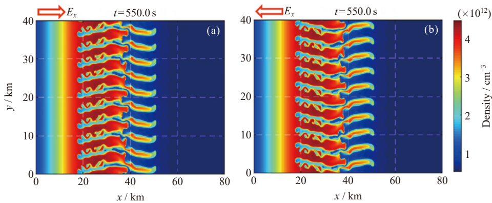
图 6 t=550 s 时不同方向背景电场 \mathbf{E}_x 作用下的等离子体密度分布
