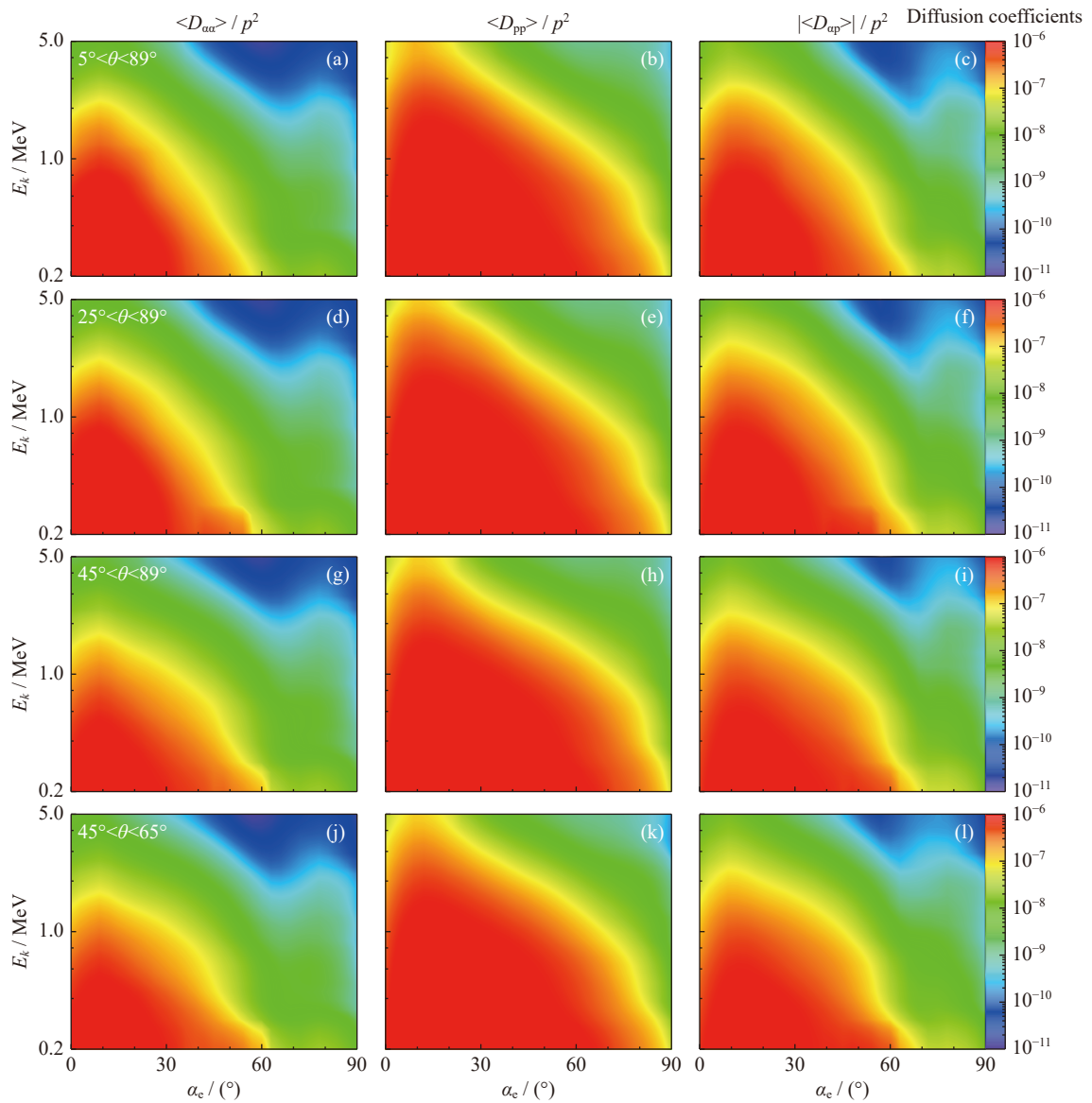
图 4 不同传播角分布的投掷角（左）、动量（中）及投掷角-动量交叉（右）弹跳平均扩散系数 2D 结果
