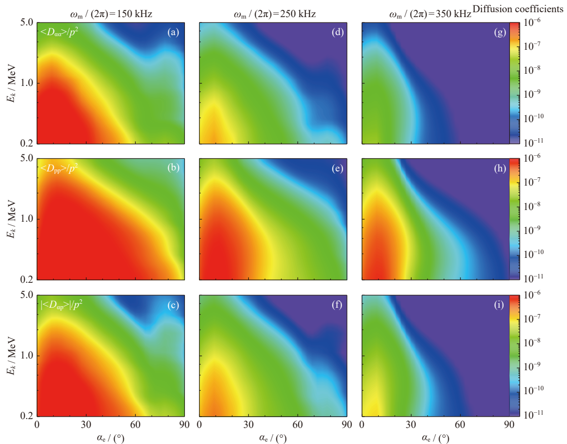
图 1 不同峰值频率的投掷角(上)、动量(中)及投掷角-动量交叉(下)弹跳平均扩散系数 2D 结果
