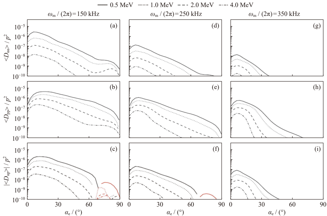
图 2 不同峰值频率的投掷角 (上)、动量 (中) 及投掷角-动量交叉 (下) 弹跳平均扩散系数 1D 结果
