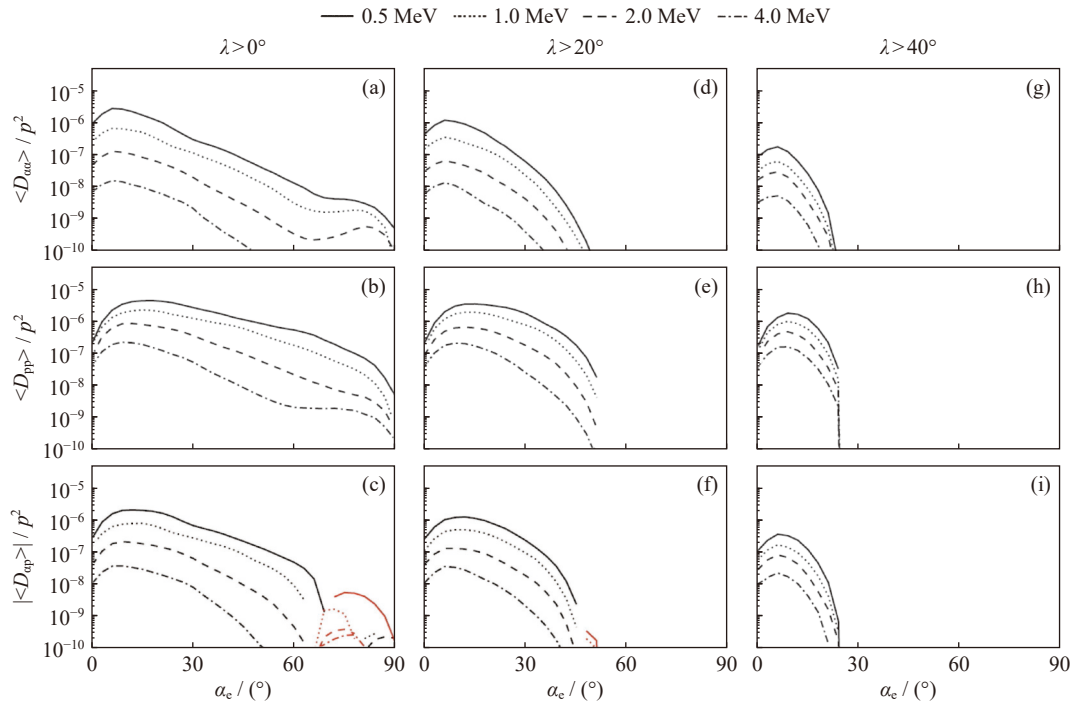
图 7 不同纬度分布的投掷角(上)、动量(中)及投掷角-动量交叉(下)弹跳平均扩散系数 1D 结果
