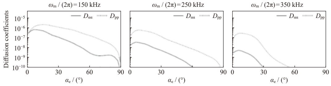
图 3 能量为 1 MeV 的投掷角扩散系数 ( D_{aa} ) 与动量扩散系数 ( D_{pp} ) 的对比
