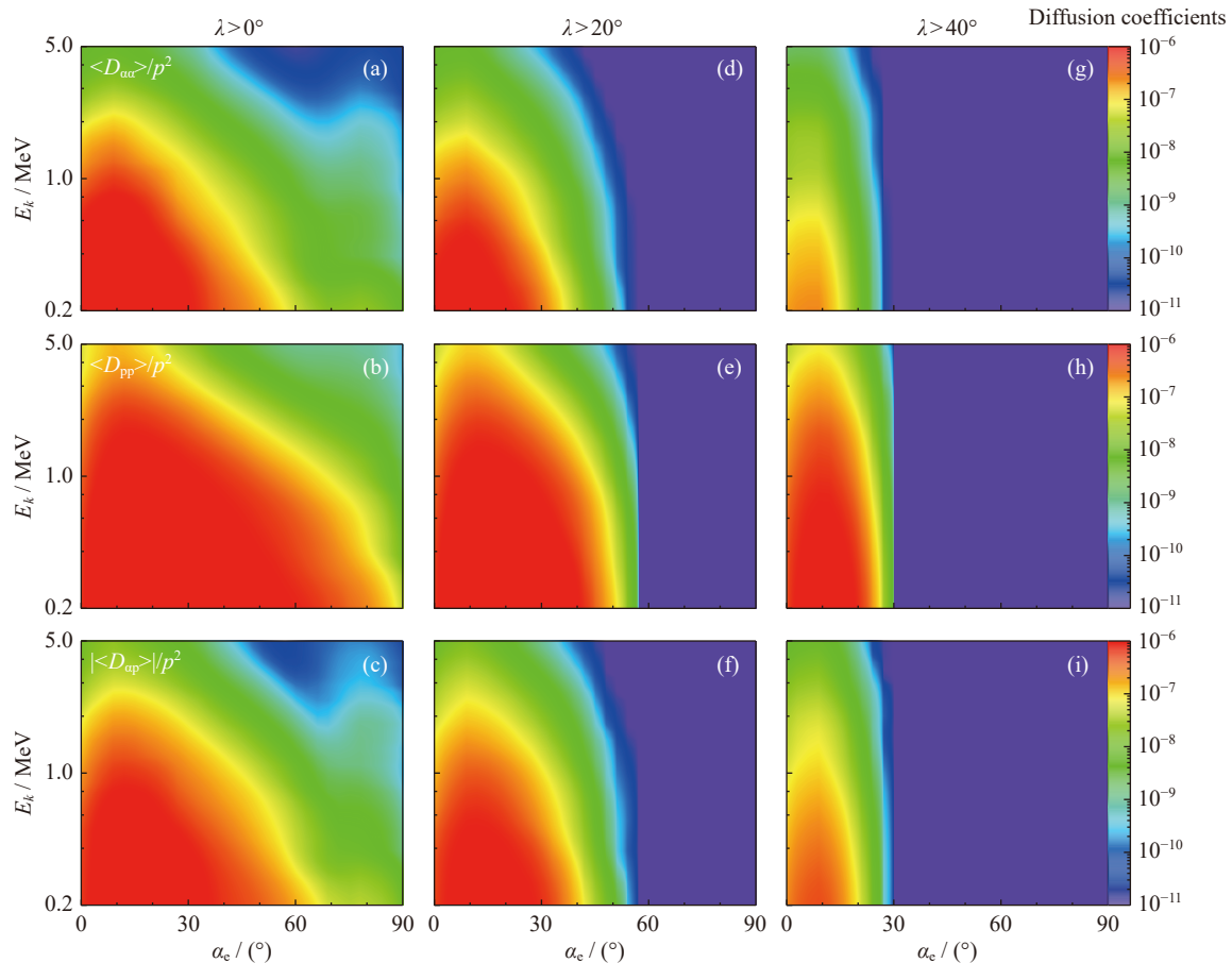
图6 不同纬度分布的投掷角(上)、动量(中)及投掷角-动量交叉(下)弹跳平均扩散系数2D结果
